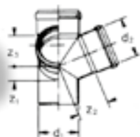
HTED – rohová odbočka 67,5°
